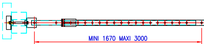
B2: Bracon bas de reprise de stab. complet (26 09 B3 60) + rallonge pour bracon bas lg 800 (26 09 C1 30)
