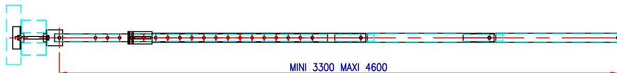
B2: Bracon bas de reprise de stab. complet (26 09 B3 60) + rallonge pour bracon bas lg 800 (26 09 C1 30)
